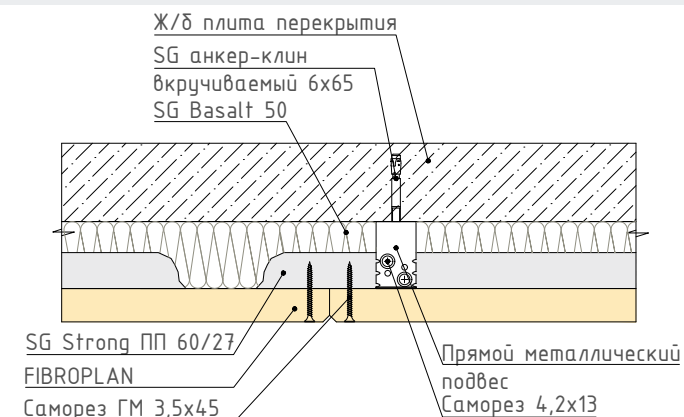
Узел крепления панели FIBROPLAN к металлическому одноуровневому каркасу
