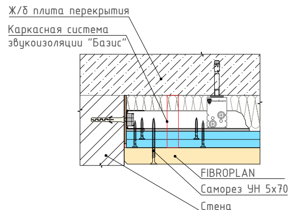
Узел крепления панели FIBROPLAN к системе звукоизоляции потолка
