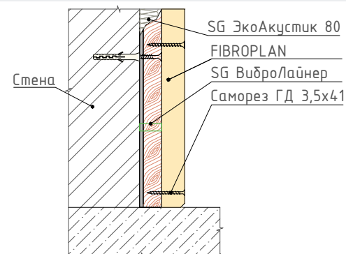
Узел крепления панели FIBROPLAN к деревянному каркасу
