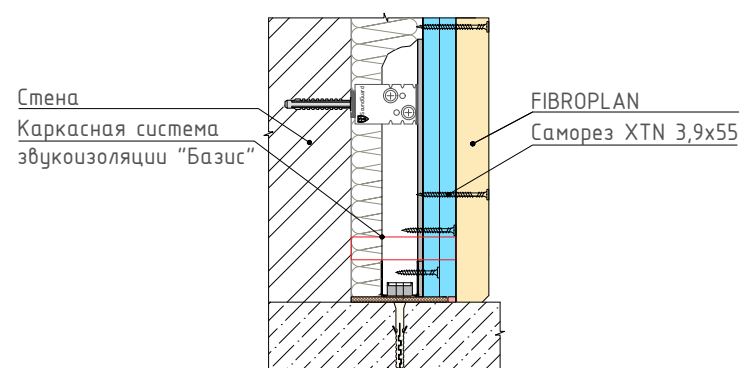
Узел крепления панели FIBROPLAN к каркасной системе звукоизоляции стены
