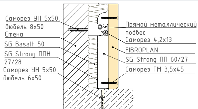
Узел крепления панели FIBROPLAN к металлическому каркасу
