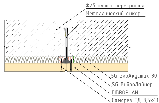
Узел крепления панели FIBROPLAN к системе звукоизоляции потолка
