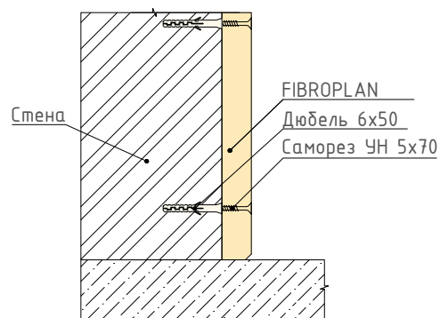
Узел крепления панели FIBROPLAN к стене бескаркасным способом
